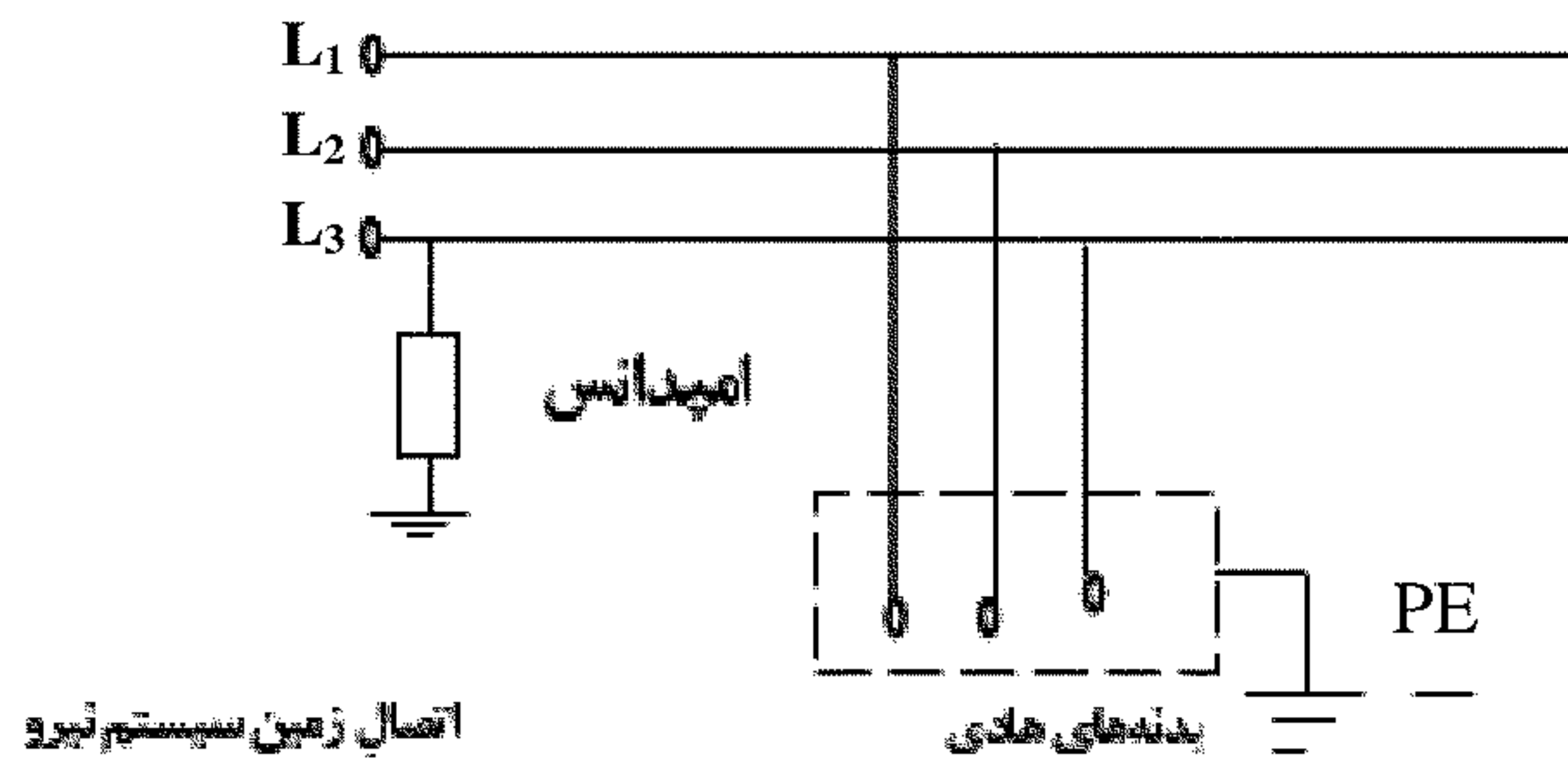
شکل پ ۵ سیستم TT
