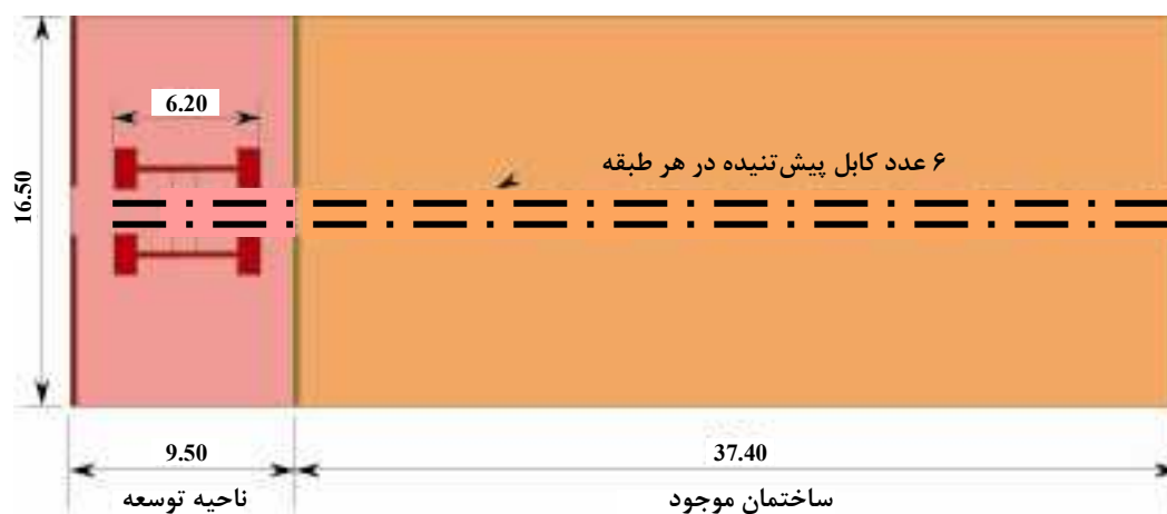
پلان کف طبقات. وضعیت موجود (راست) و بخش توسعه جدید (چپ) که توسط دیوار بتن مسلح I شکل مهار شده است.
