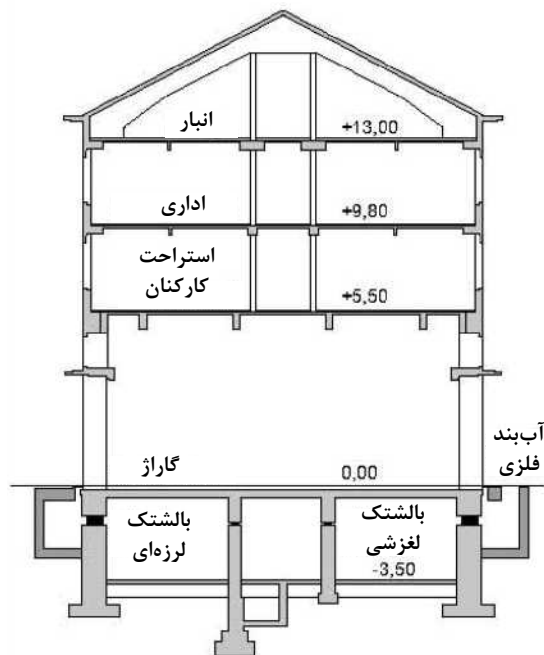
مقطع عرضی ساختمان به همراه بالشتک‌های لرزه‌ای در زیرزمین (بچمن و زچمن، ۲۰۰۸)
