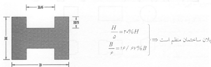
شکل ۱-۳۶- ضوابط فرورفتگی یا پیش‌آمدگی در پلان‌های منظم
