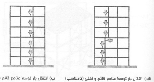
الف) انتقال بار توسط عناصر قائم و افقی (نامناسب) ب) انتقال بار توسط عناصر قائم (مناسب)
